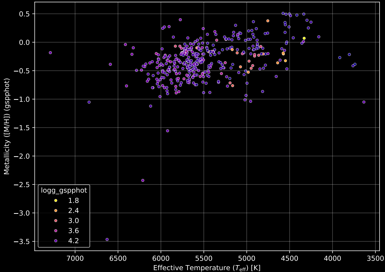
GALAH DR4 Field: [6695] Stellar Population Parameters (n= 377)
