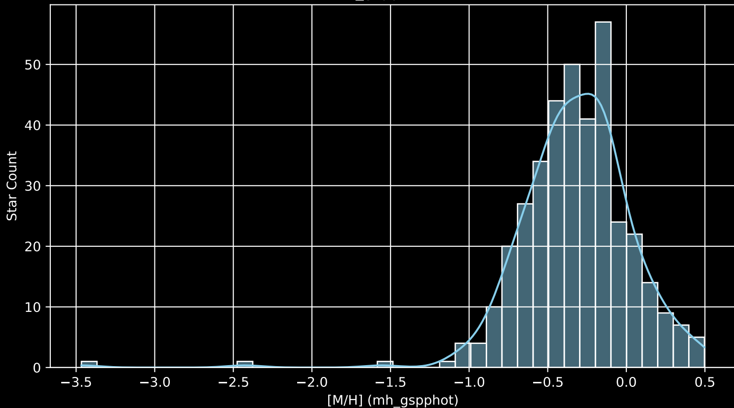
GALAH DR4 Field: [6695] [M/H] (mh_gspphot) (n= 376)
