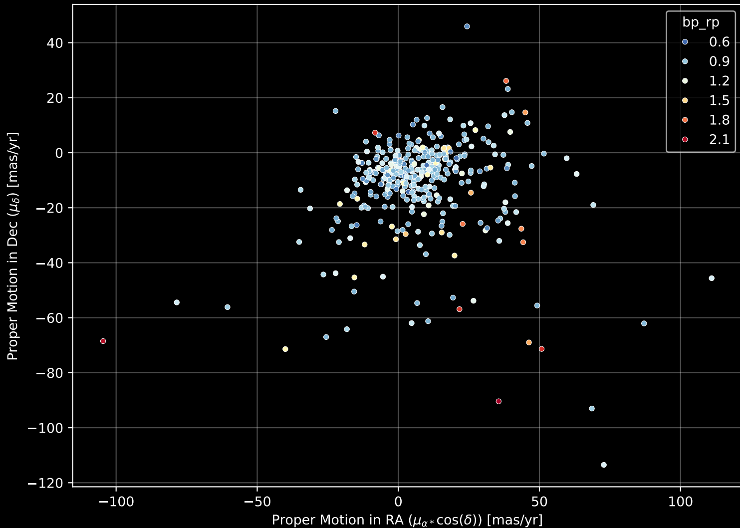
GALAH DR4 Field: [6695] Proper Motion Diagram (n= 377)
