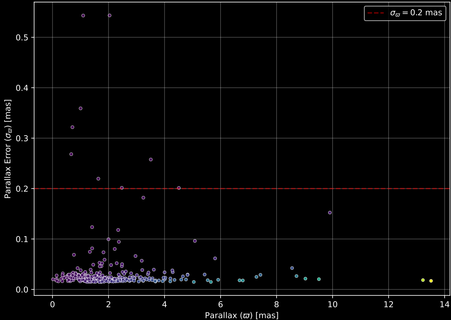
GALAH DR4 Field: [6695] Parallax Quality (n= 377)
